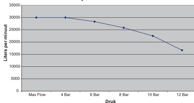
Capaciteitscurve
