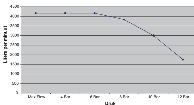
Capaciteitscurve
