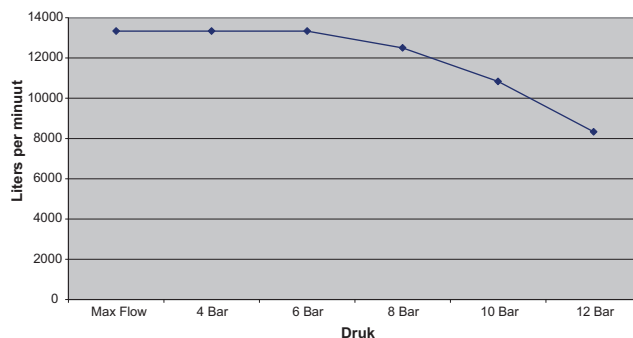
Capaciteitscurve
