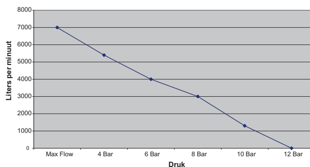
Capaciteitscurve
